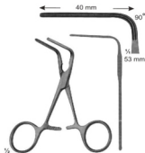
17-174 DE-BAKEY 90° winklig gebogen angled 90° 105 mm
